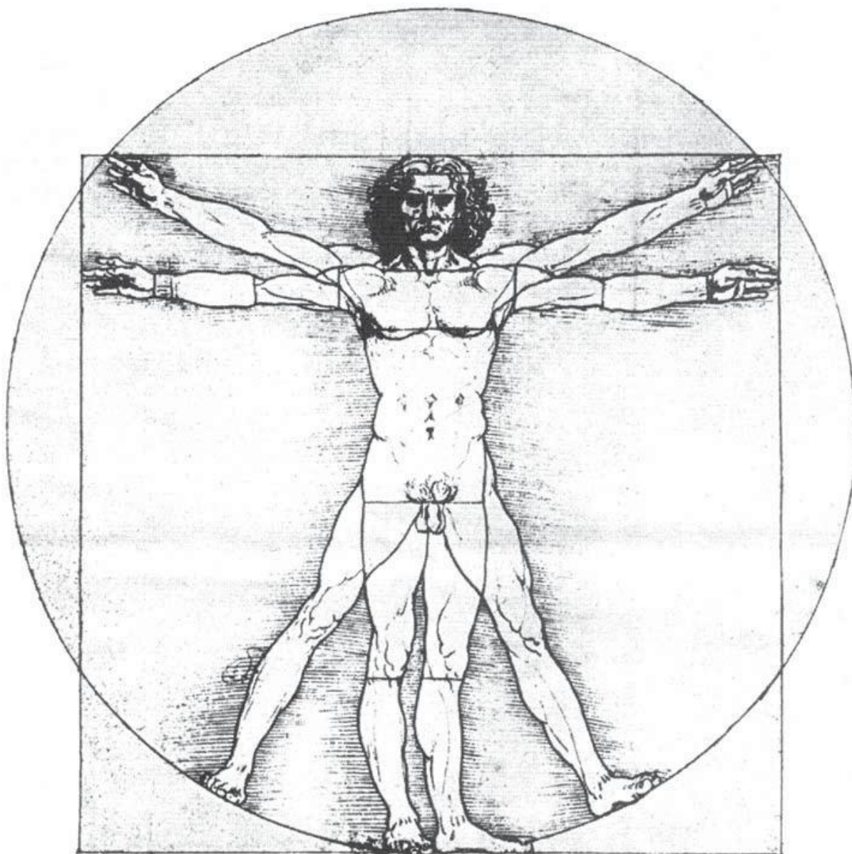
Figura 9 A retratação do Homem de Leonardo da Vinci de acordo com a geometria sagrada conhecida como Relação de Ouro.
