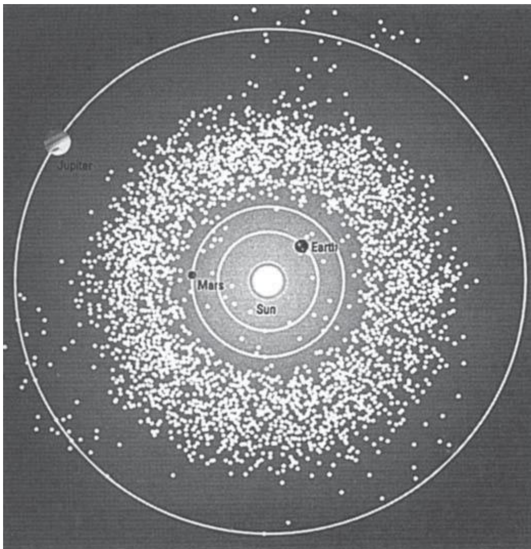
Figura 2 O Sistema Solar mostrando a localização do cinturão de asteróides entre Marte (Marte) e Júpiter, que embora os detalhes variem, muitos registros antigos e modernos sugerem ser este cinturão os restos de um planeta ou parte de um planeta.
