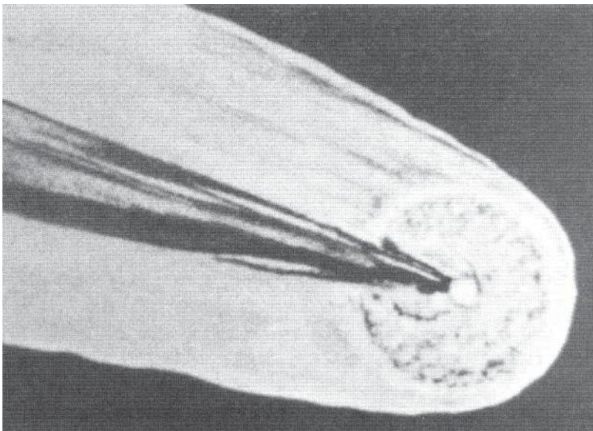
Figura 23: Um desenho do cometa de Donati em 1854 mostrando como a massa em desintegração é lançada para fora por uma força centrífuga, para “orbitar” uma fonte central de energia. Isto deixa o interior oco, do mesmo modo, que a roupa gira em torno de uma cavidade vazia numa máquina de lavar ou de secar centrífuga. Com certeza isso deve ter acontecido também quando a Terra estava se formando?
